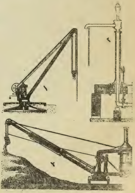
۱ - قول ايله متحرك ۲ - قضيه ماه ايله ۳ - بخارايله متحرك . ( ماچونه )
